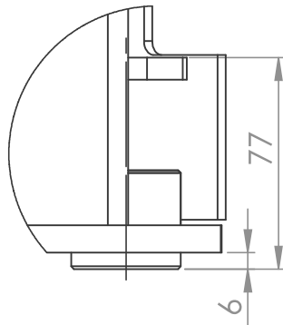
SZCZEGÓŁ B SKALA 2 : 5
