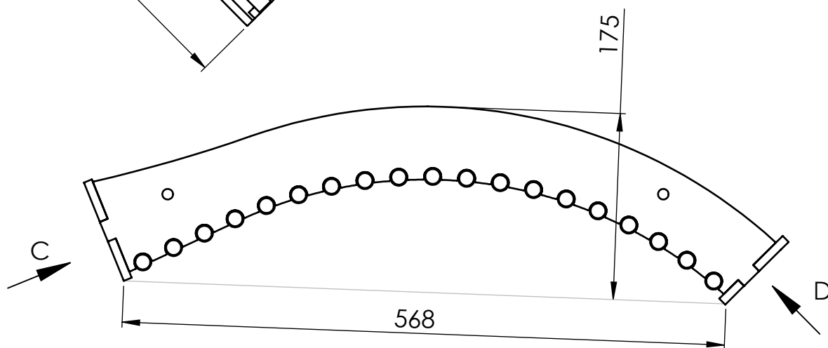
WIDOK D
