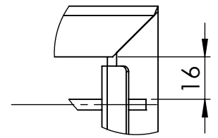
SZCZEGÓŁ C SKALA 1 : 2
