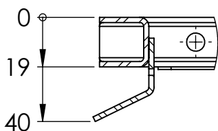
SZCZEGÓŁ E SKALA 1 : 2
