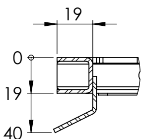
SZCZEGÓŁ C SKALA 1 : 2
