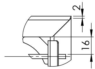
SZCZEGÓŁ E SKALA 1 : 2
