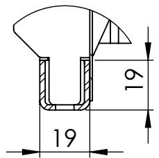
SZCZEGÓŁ D SKALA 1 : 2
