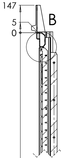
SZCZEGÓŁ B
