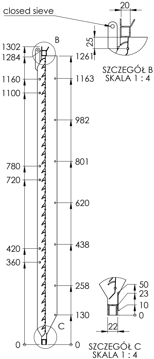
PRZEKRÓJ A-A
