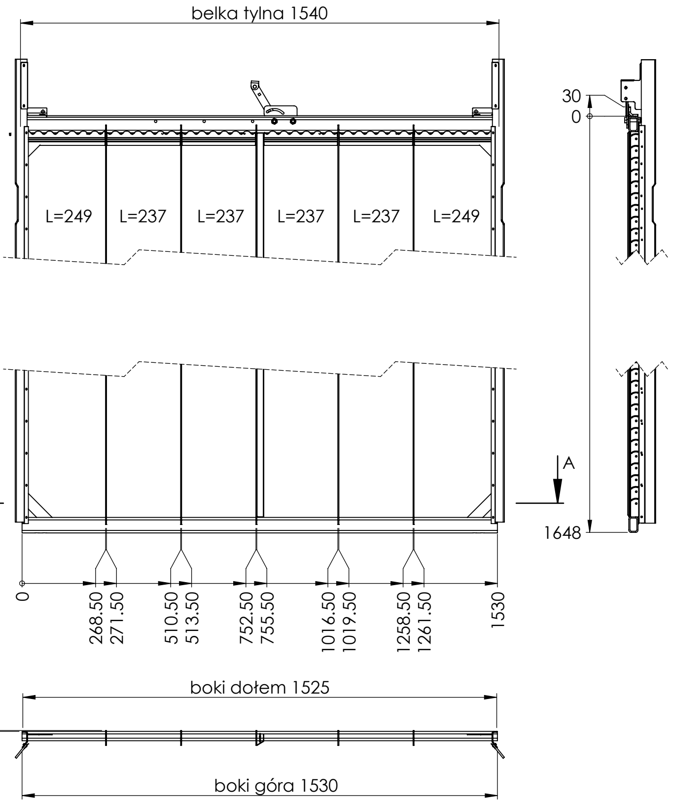
PRZEKRÓJ A-A
